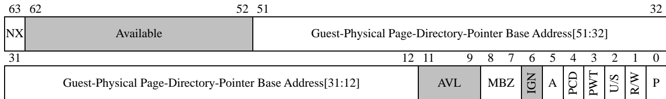
Figure 37: AMD64 Long Mode 1-Gbyte PML5E Format
