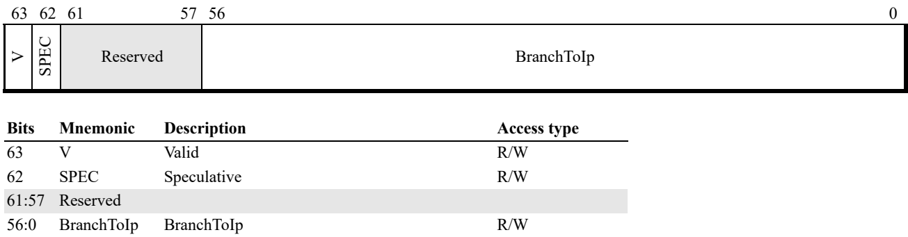
Figure 13-8. LastBranchStackToIp MSR
