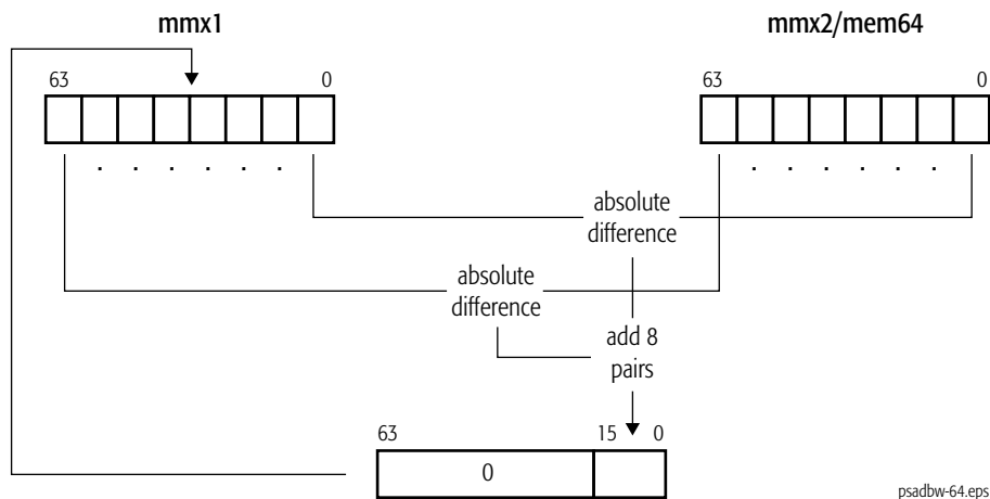
psadbw-64.eps
