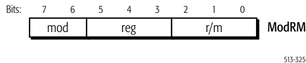
Figure A-1. ModRM-Byte Fields
