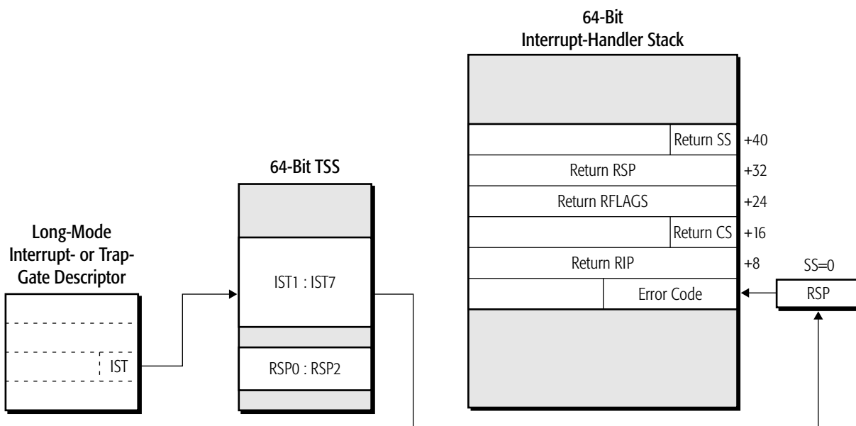
Figure 8-16. Long-Mode IST Mechanism
