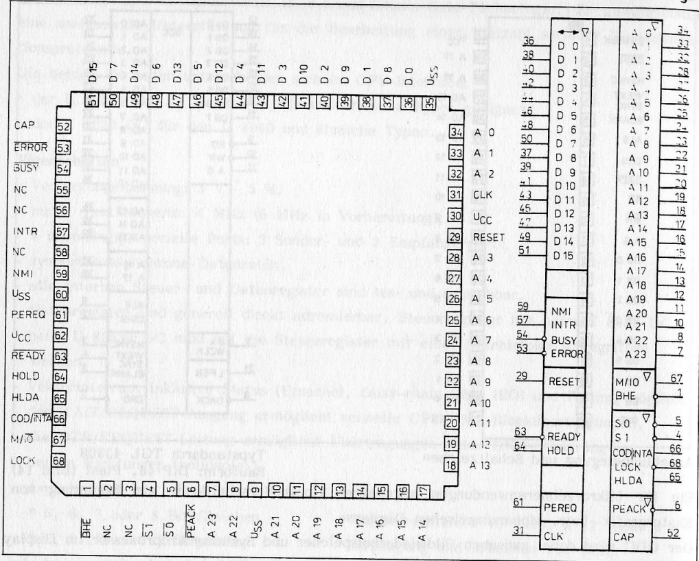
Anschlußbelegung und Schaltzeichen
