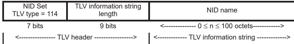
Figure 11-20—NID Set TLV format
